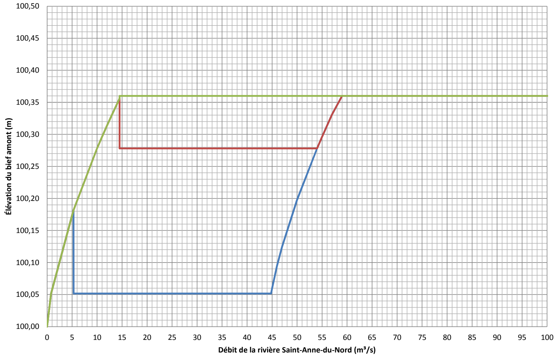
Figure A-2 : Courbe de tarage du bief amont (2/2)
